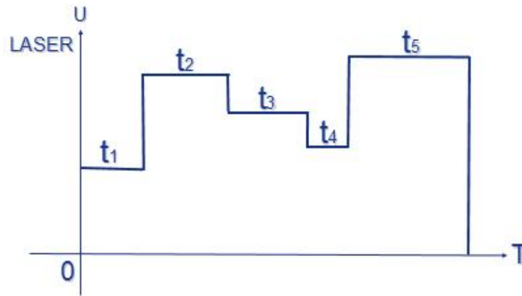
图 2-4 五段编程波形显示
